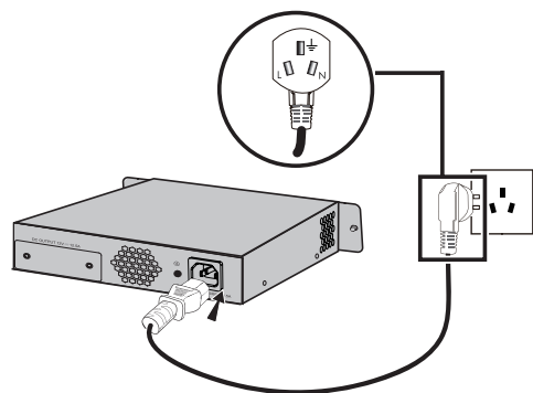
图3-6 TL-RPS200连接电源线示意图
